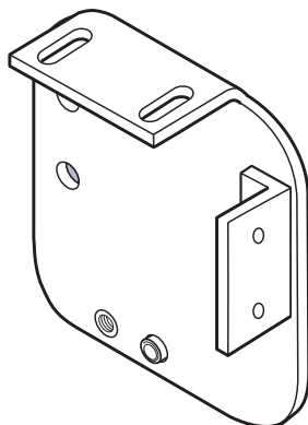
Vrchní připevňovací konzole
